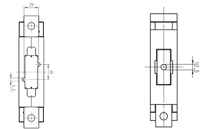
Base plate mounting Aufbaumontage
