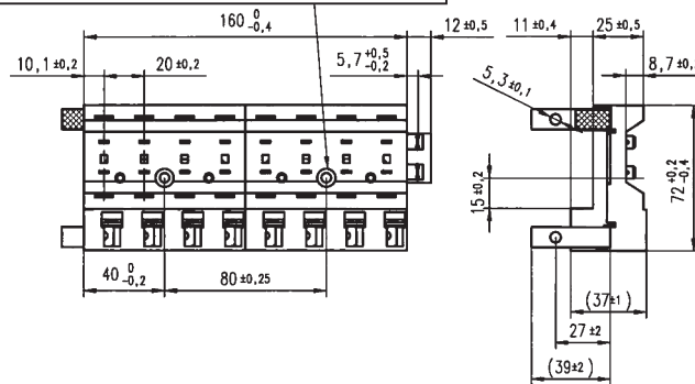
Breaker plug connector Schutzschalter Stecker
